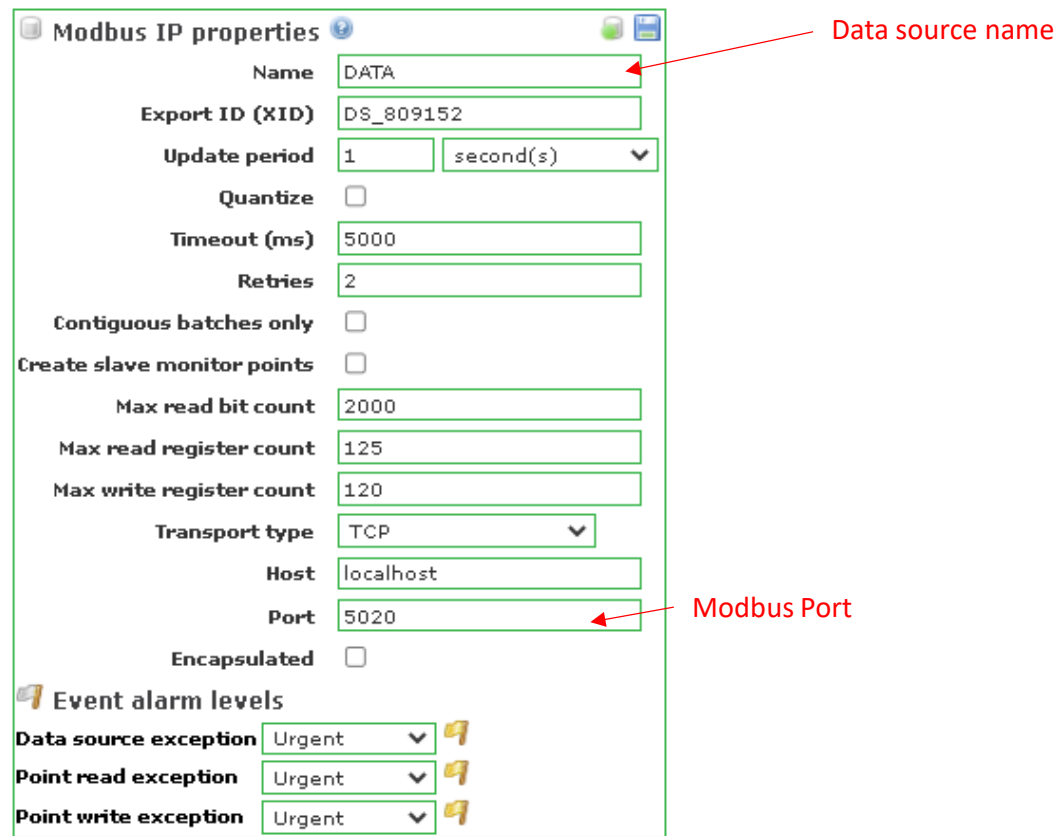
Fig. A4. Modbus IP Properties
